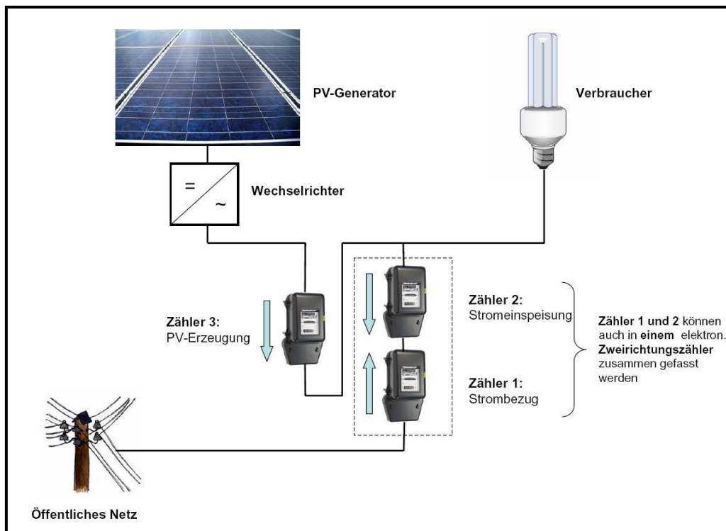
Abb. 4 Schaltschema zum Eigenverbrauch im Einfamilienhaus
